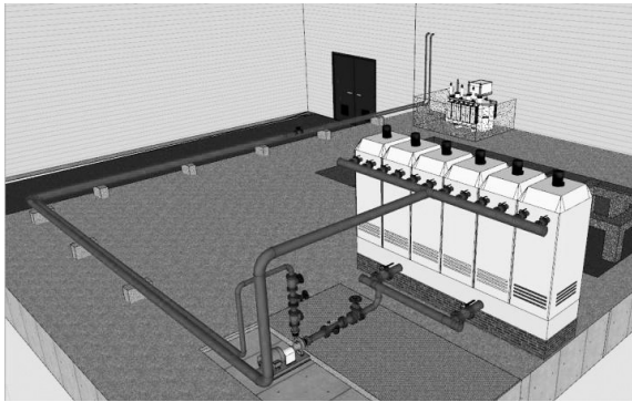
Figura 1 - Representação das torres de refrigeração e bomba do sistema de distribuição de água de refrigeração, parte externa Fonte: Autores, (2010).
