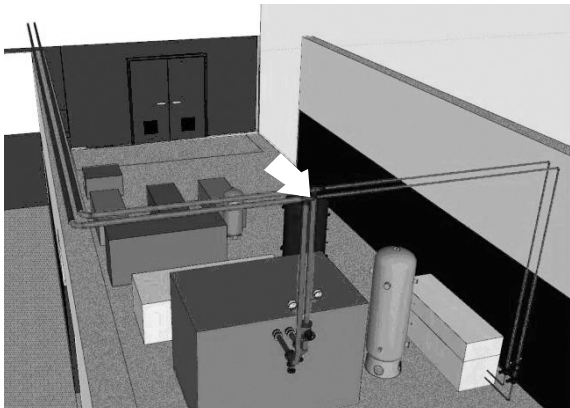
Figura 2 - Sistema interno de distribuição de água. A bifurcação que divide os escoamentos está assinada com uma flecha. Logo abaixo está o compressor e, à direita, o secador Fonte: Autores, (2010).
